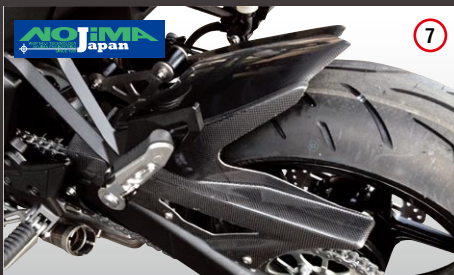
フェンダーレスとあわせて装着したいのがリアフェンダー。 ドレスアップはもちろん、純正比70mmロングで泥はねも しっかりガードします。
