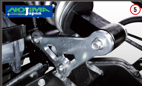
NOJIMAロゴ入り アルミ削り出し サイズは純正同等です。
