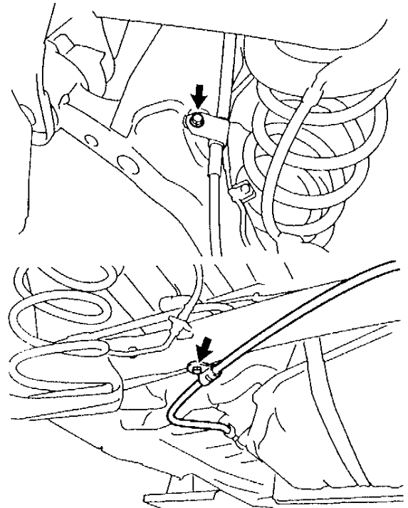
サイドブレーキワイヤークランプ部
