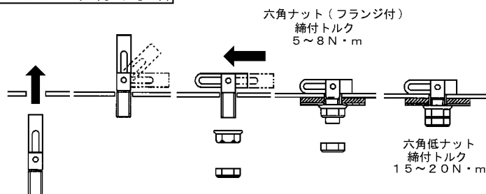
ITボルト組付け手順
