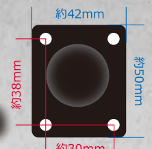
寸法図
