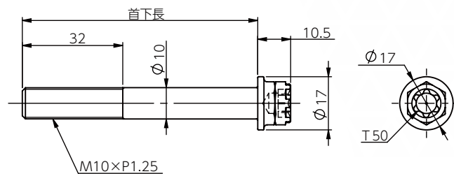
フランジ六角ボルト寸法図
