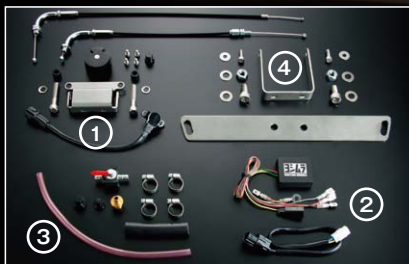
キャブコンバージョンキット セット内容
