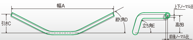
ハンドル寸法図
